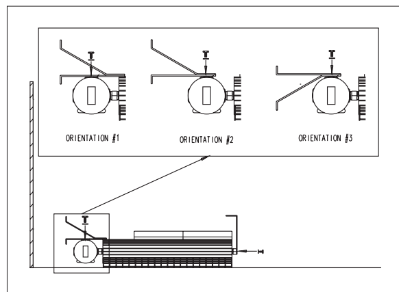
Figure 7 – Installation du support de fixation sur le radiateur
