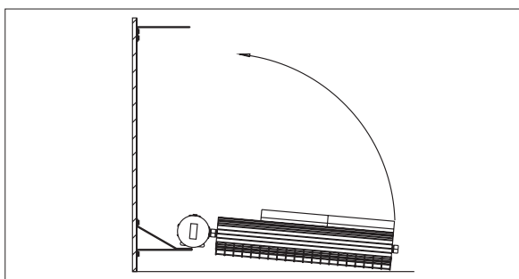
Figure 4 – Schéma de fixation au mur
