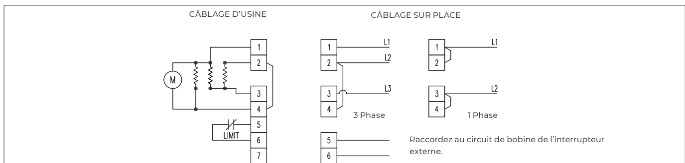
Figure 3A – Schéma de raccordement des appareils de la série GE de 2 à 10 kW avec option de limite élevée. Modèles de 208 V et 210 V.
