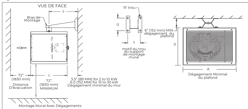
Figure 2 – Dégagement d'installation
