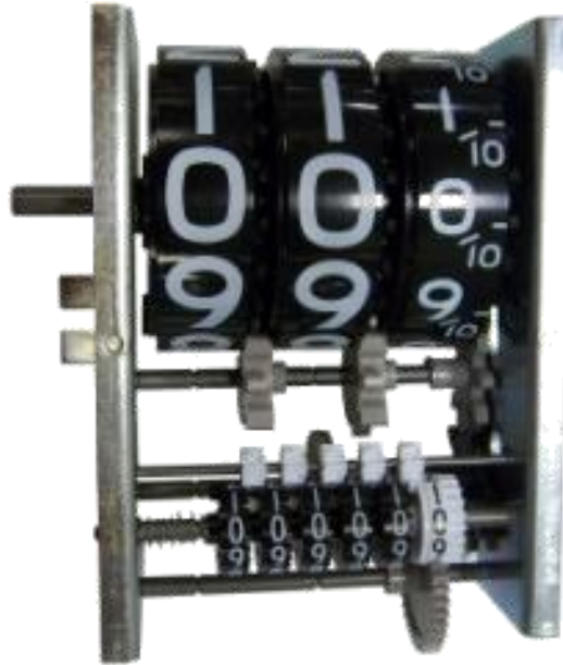
Gallon Register (5)
